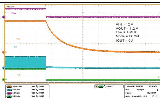
图 26. Shutdown Operation
