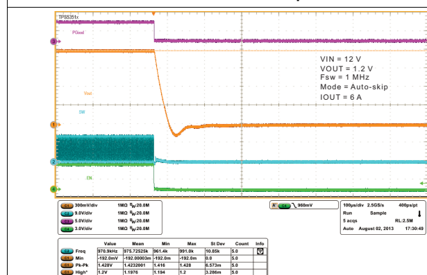
图 27. Shutdown Operation
