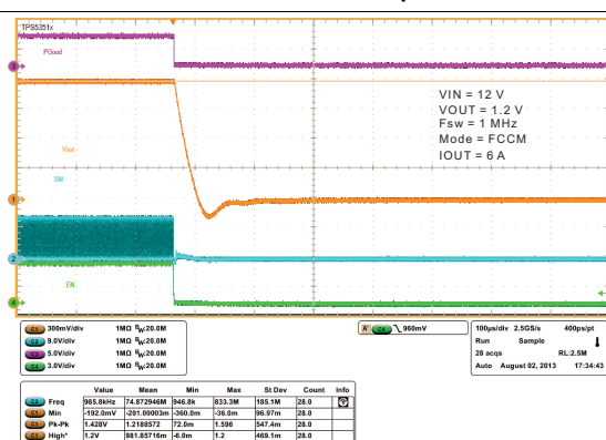
图 28. Shutdown Operation
