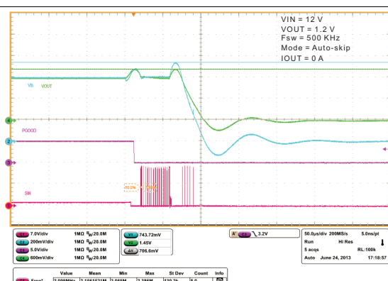
图 30. Overvoltage Protection
