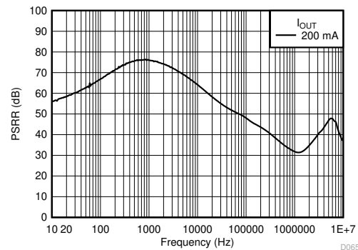
图 7-6. PSRR
