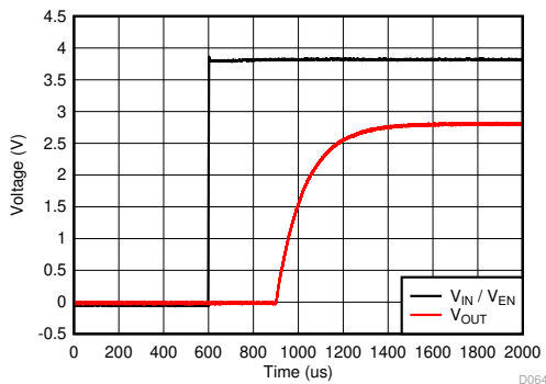
图 7-5. Start-Up
