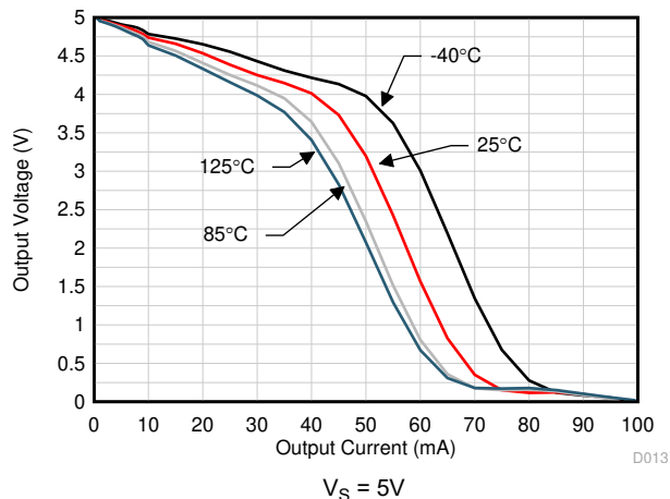
图 6-13. 输出电压摆幅与输出电流 (拉电流) 间的关系
