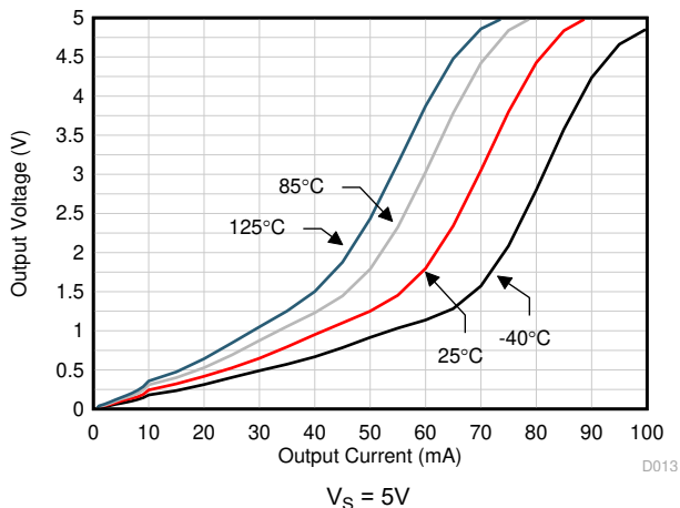
图 6-14. 输出电压摆幅与输出电流 (灌电流) 间的关系
