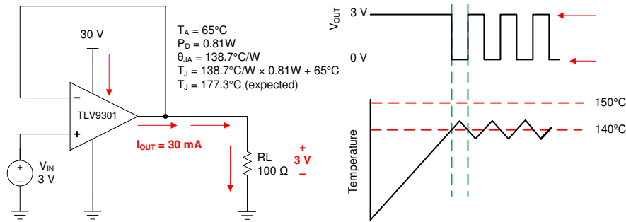
图 7-5. 过热保护
