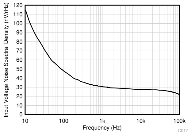
图 6-19. 输入电压噪声频谱密度与频率间的关系
