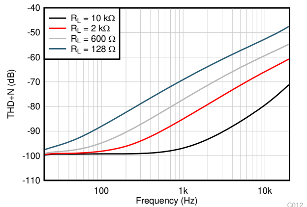
图 6-20. THD+N 比与频率间的关系
