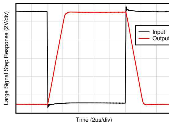
图 6-34. 大信号阶跃响应 (下降)
