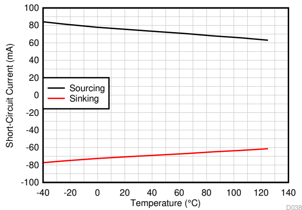
图 6-37. 短路电流与温度间的关系
