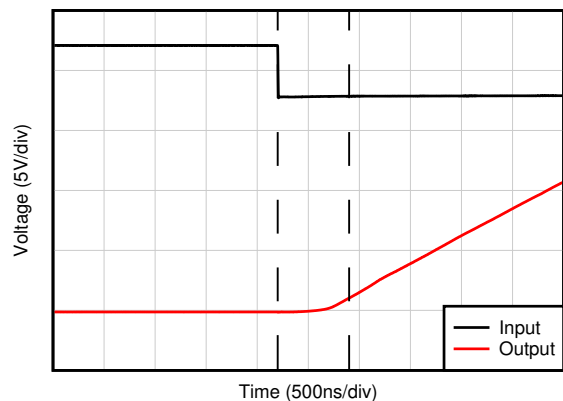
图 6-31. 负过载恢复
