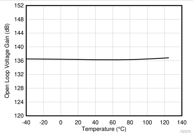
图 6-24. 开环电压增益与温度间的关系 (dB)
