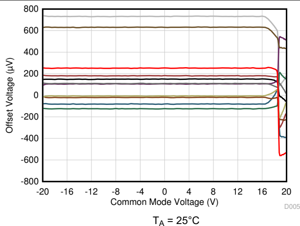
图 6-5. 失调电压与共模电压间的关系
