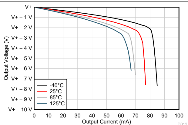
图 6-11. 输出电压摆幅与输出电流 (拉电流) 间的关系
