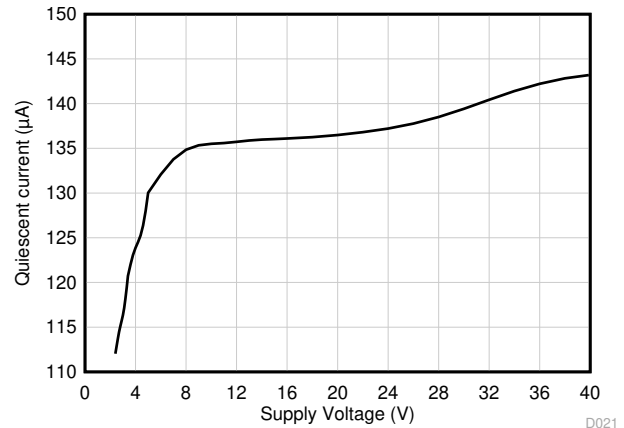
图 6-22. 静态电流与电源电压间的关系
