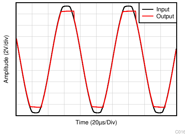
图 6-29. 无相位反转
