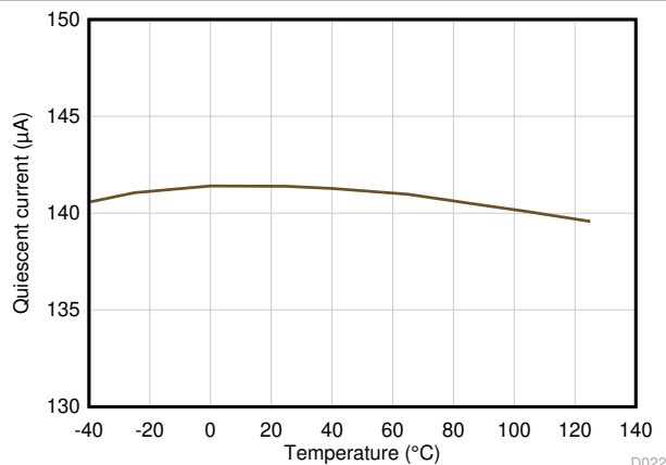
图 6-23. 静态电流与温度间的关系
