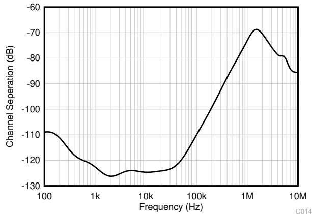
图 6-39. 通道隔离与频率间的关系
