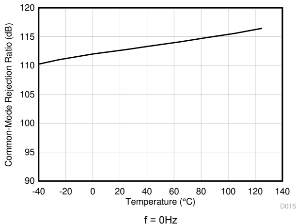
图 6-16. CMRR 与温度间的关系 (dB)
