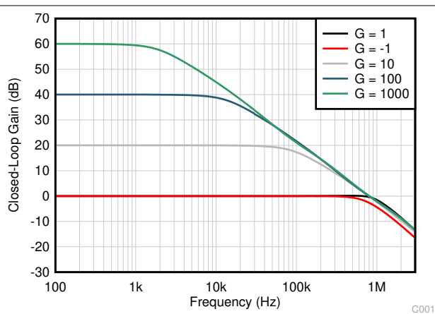
图 6-8. 闭环增益和相位与频率间的关系
