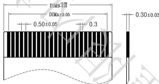
适用扁平线
