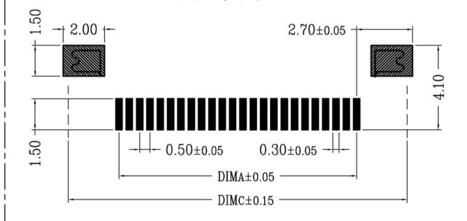
适用线路板
