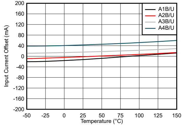
图 7-2. TMCS1107-Q1 输入失调电流与温度间的关系
