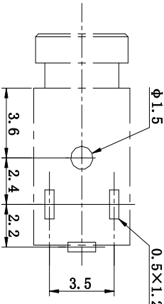
印制线路板开孔尺寸
