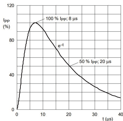
IEC 61000-4-5 Waveform( 8/20 \mu\text{s} pulse)
