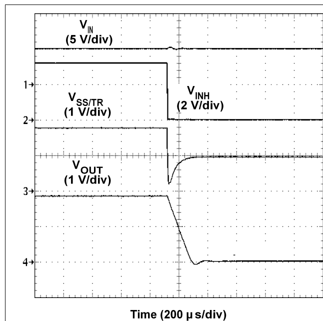
图 31. Inhibit Turn-Off
