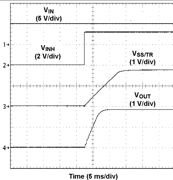
图 32. Inhibit Turn-On
