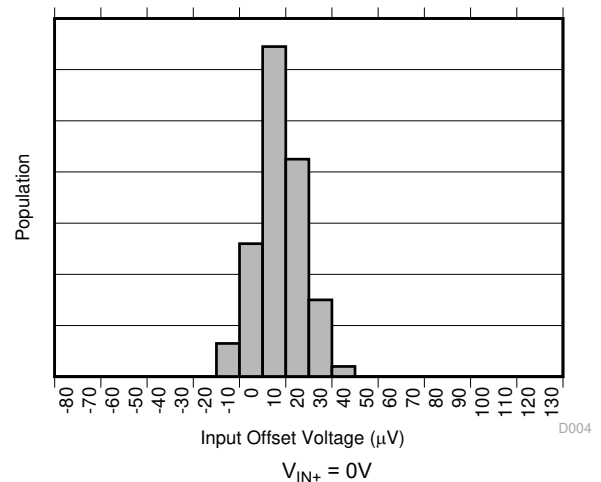
图 7-4. 输入失调电压产生分布图 A4
