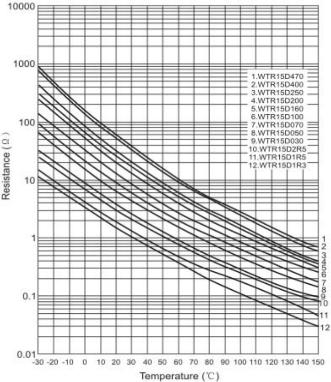
10.2溫度－電阻特性
