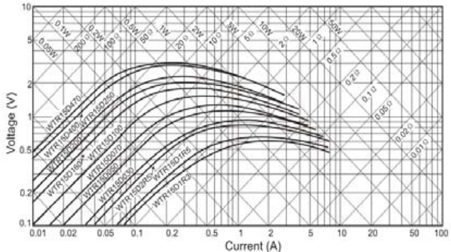
10.4電流－電壓特性
