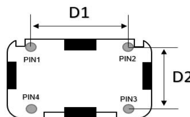
底视图 bottom view
