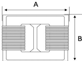
正视图 front view
