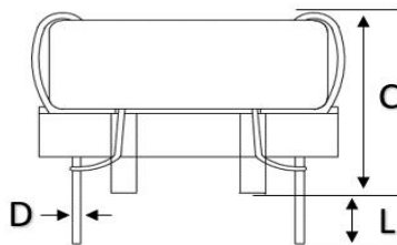
側视图 side view
