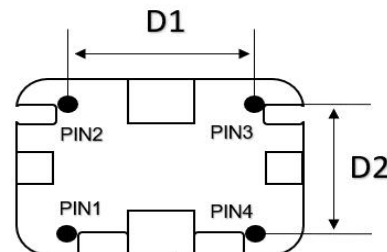
底视图 bottom view
