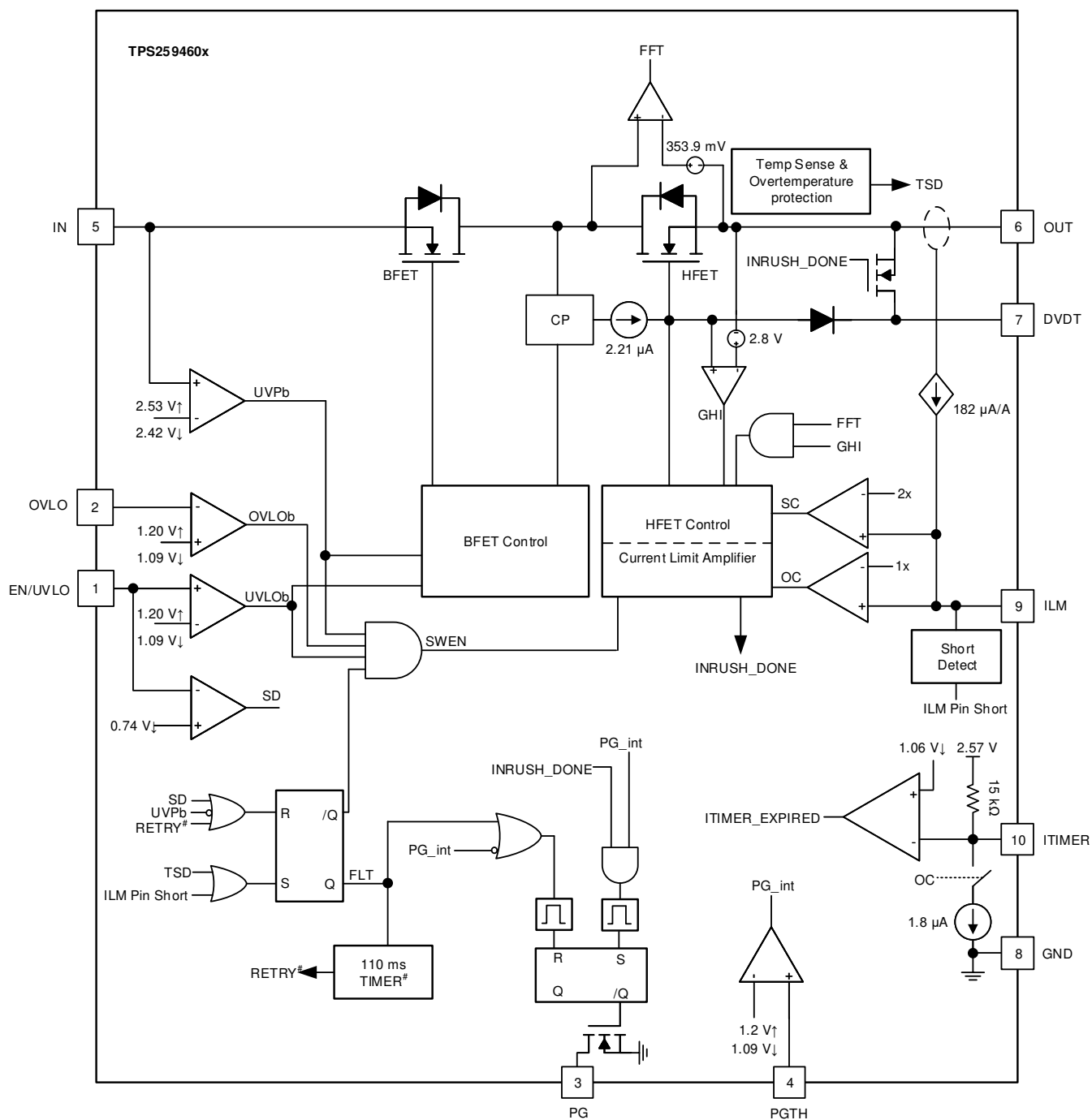
图 8-1. TPS25946x Block Diagram
