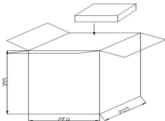
外包装尺寸图
