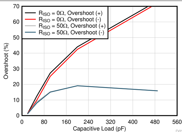
图 6-5. 小信号过冲与容性负载之间的关系 ( 20\text{mV}_{pp} 输出阶跃, G = +1 )
