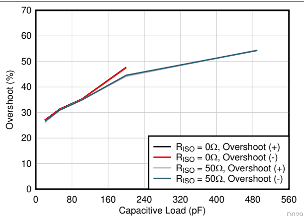
图 6-6. 小信号过冲与容性负载之间的关系 ( 20\text{mV}_{pp} 输出阶跃, G = -1 )
