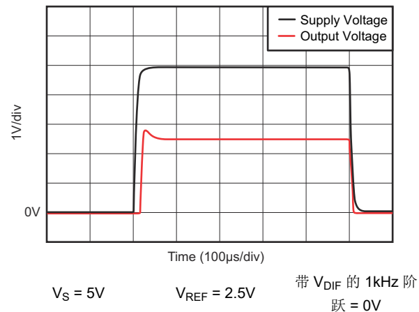
图 5-21. 启动响应
