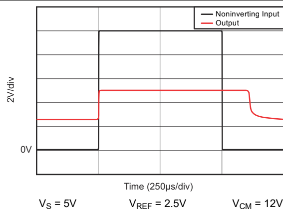
图 5-20. 同相差分输入过载
