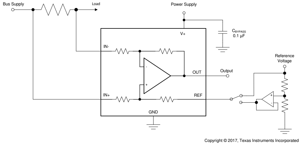
图 7-3. 双向应用原理图
