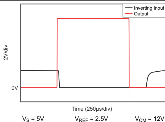
图 5-19. 反相差分输入过载
