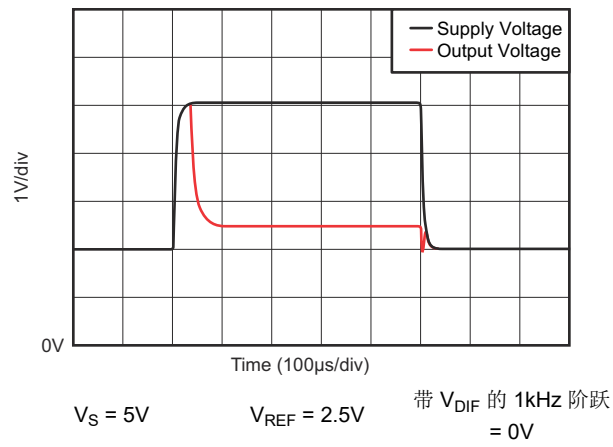
图 5-22. 欠压恢复
