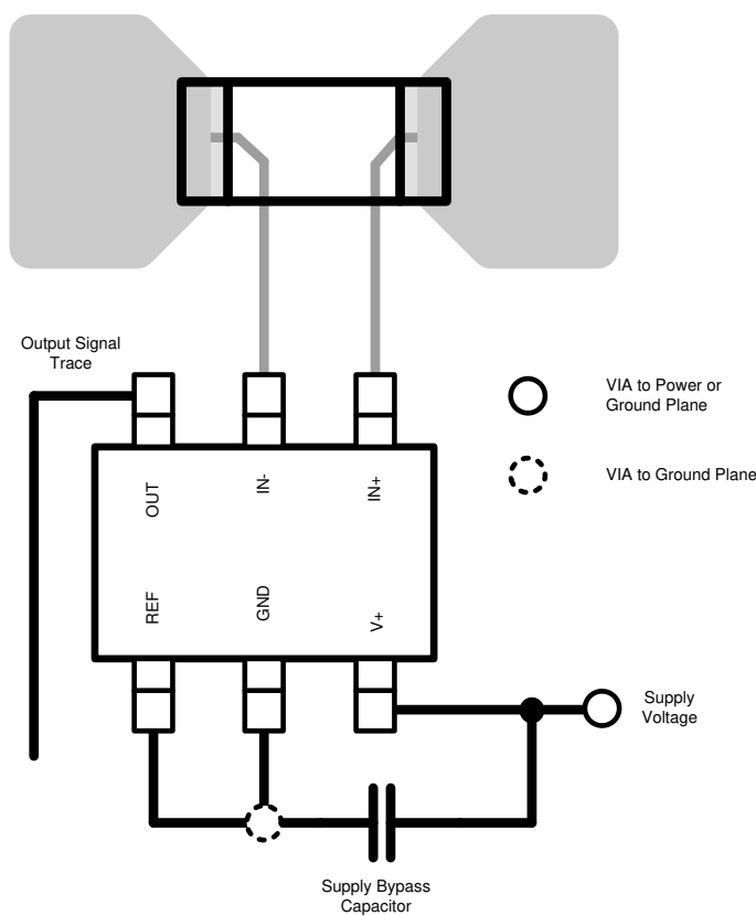
图 9-1. 建议布局
