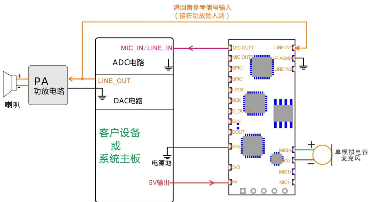
单模拟麦克风连接图（消回音模式一）
