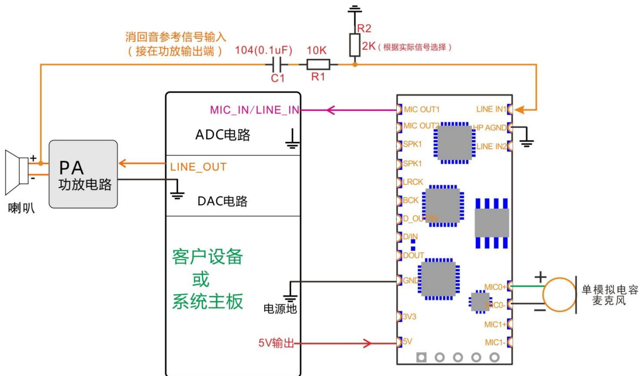
单模拟麦克风连接图（消回音模式二）
