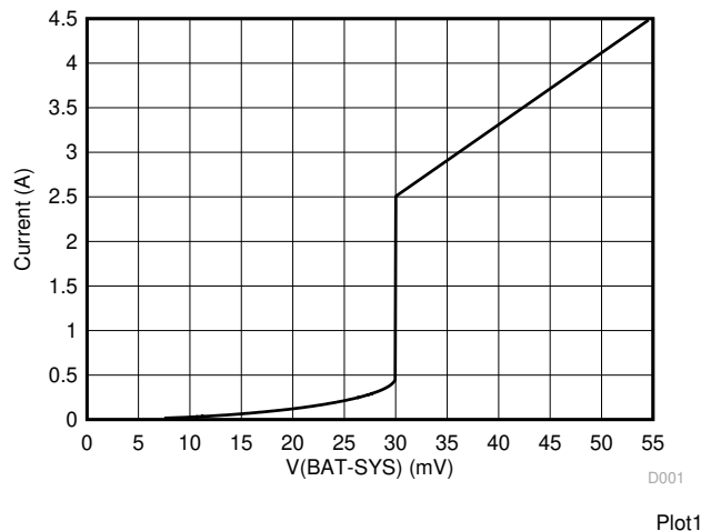
图 9-9. BATFET V-I Curve
