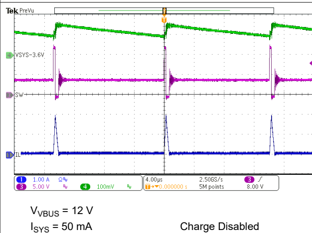
图 10-6. PFM Switching in Buck Mode
