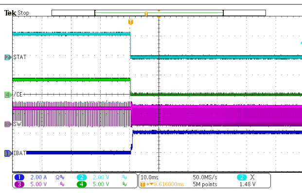
图 10-9. Charge Enable
