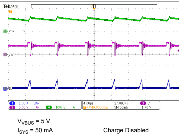
图 10-4. PFM Switching in Buck Mode
