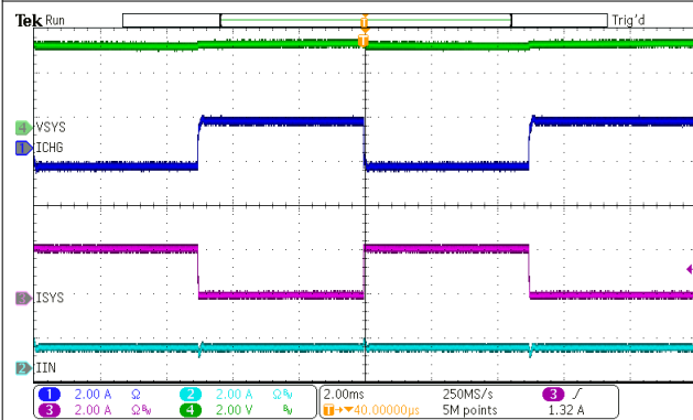
图 10-14. System Load Transient
