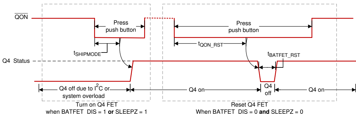
图 9-10. QON Timing
