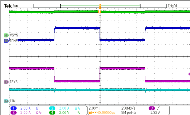
图 10-16. System Load Transient
