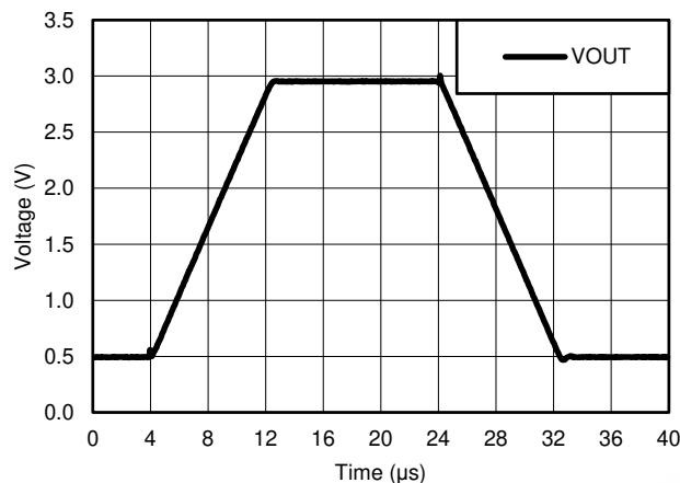
图 5-43. 电压跟随器大信号脉冲响应 (50pF)
