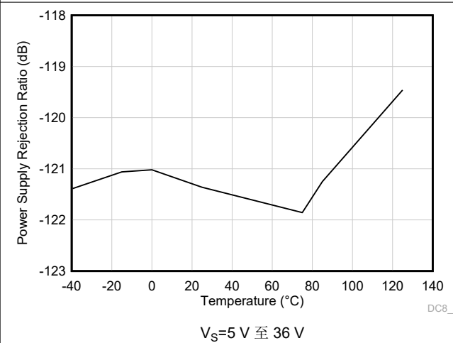
图 5-15. 电源抑制比与温度间的关系 (dB)
