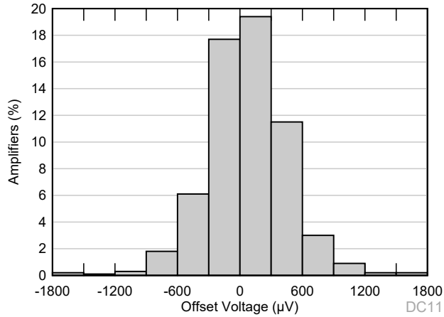
图 5-1. 失调电压生产分配
