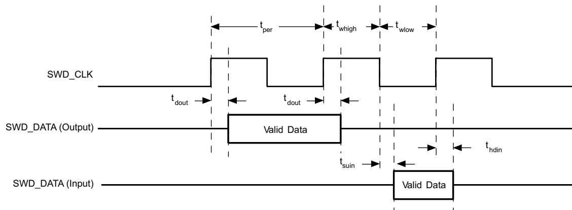
图 7-6. SWD Timing
