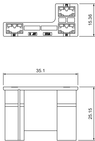
RSFP-3V-ES-B
