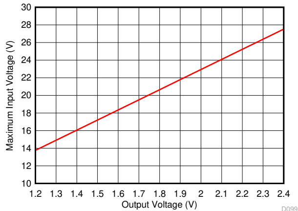
图 6-1. Maximum Input Voltage for V_{OUT} < 2.5\text{V}
