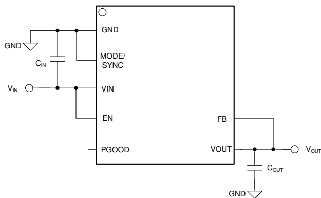
24V 至 5V、1A 直流/直流转换器的固定输出选项原理图
