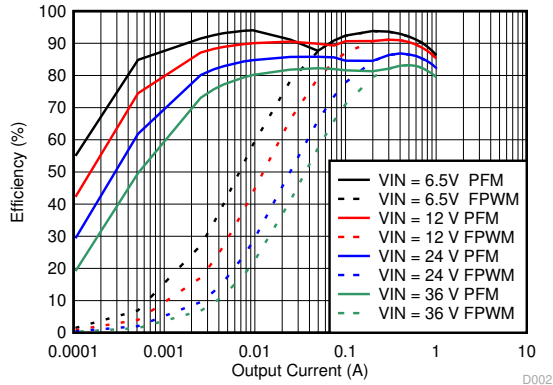
图 8-6. Efficiency
