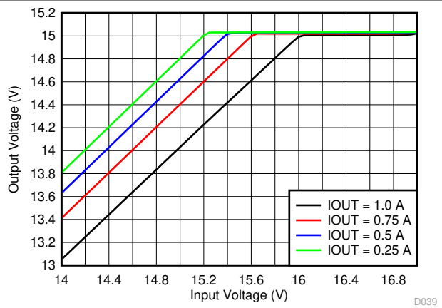
图 6-4. Dropout Voltage
