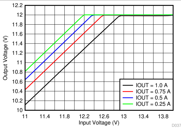
图 6-3. Dropout Voltage
