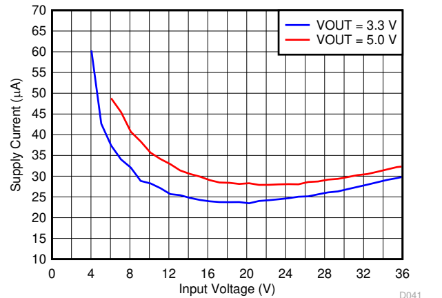
图 6-2. Input Supply Current
