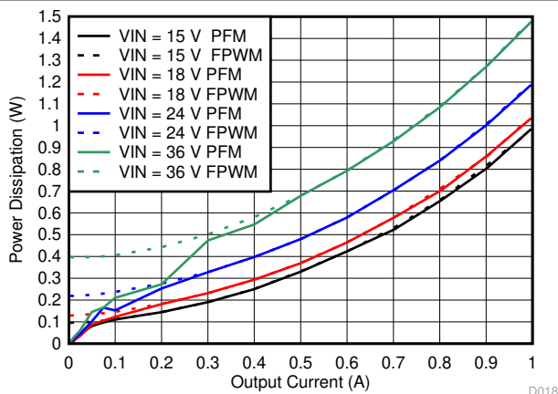
图 6-11. Power Dissipation
