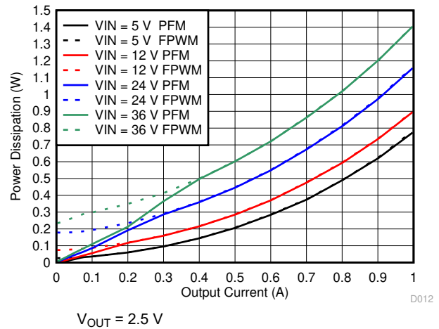
图 6-14. Power Dissipation
