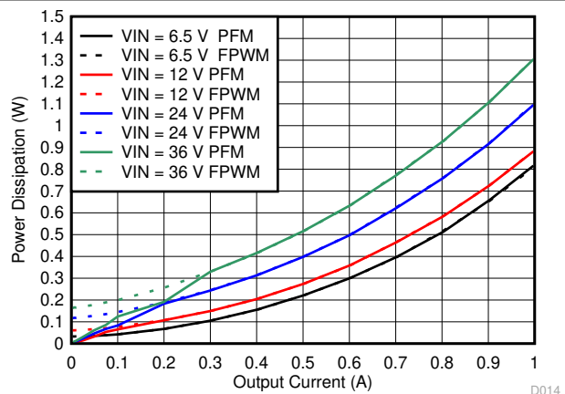
图 6-10. Power Dissipation
