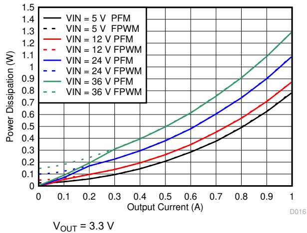
图 6-13. Power Dissipation
