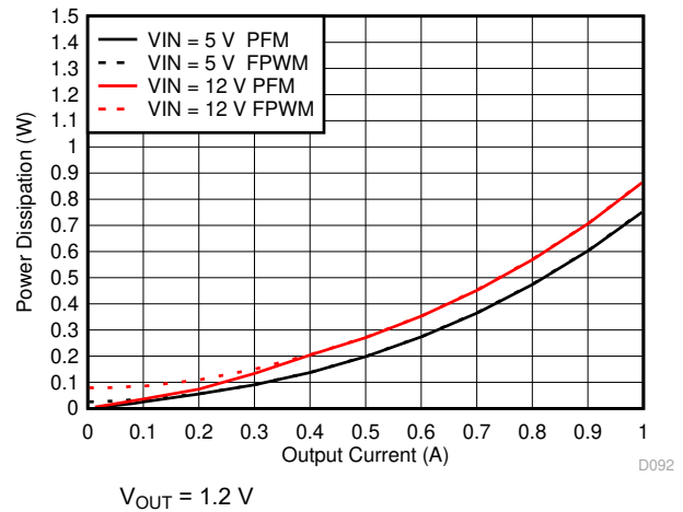
图 6-16. Power Dissipation
