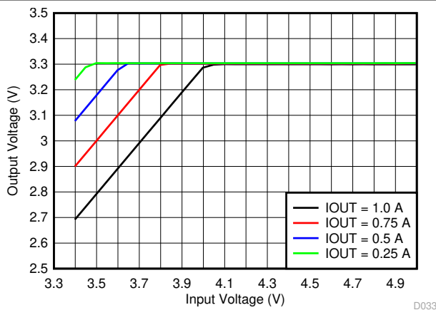
图 6-3. Dropout Voltage
