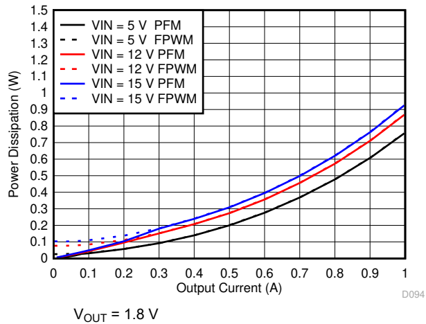
图 6-15. Power Dissipation
