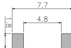
PCB. 焊接图
