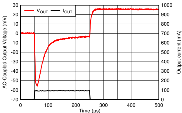
图 6-56. Load Transient
