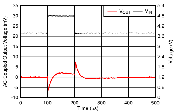
图 6-33. Line Transient
