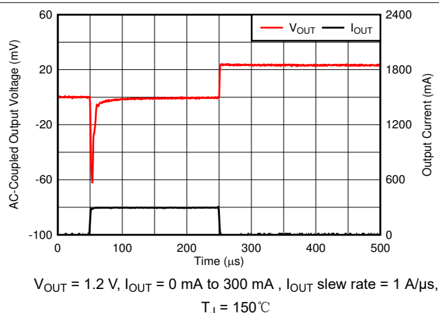
图 6-52. Load Transient
