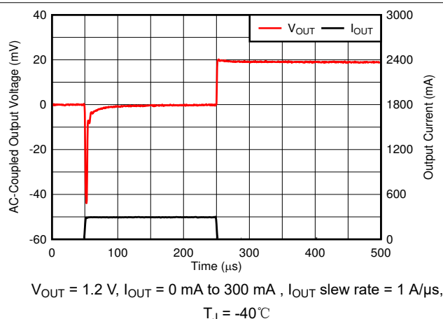
图 6-51. Load Transient
