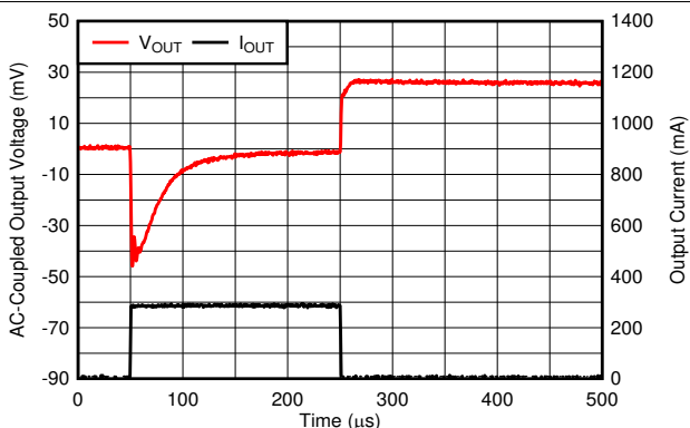
图 6-58. Load Transient
