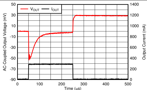
图 6-57. Load Transient
