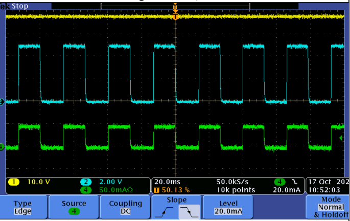
Fig 6. V_{IN}=36V , V_{OUT}=5V , R_{LOAD}=100\Omega , 热保护
