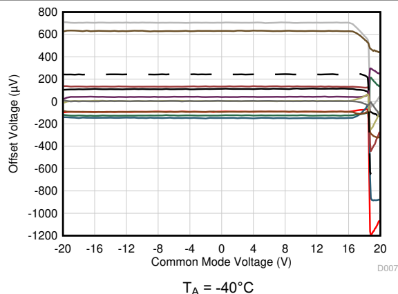
图 6-8. 失调电压与共模电压间的关系
