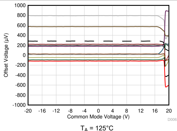
图 6-7. 失调电压与共模电压间的关系
