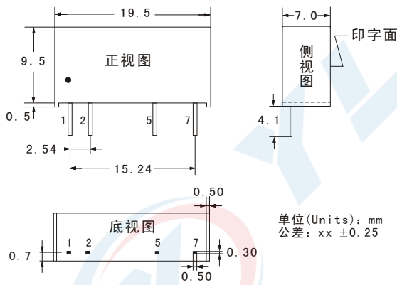
1) 外观尺寸
