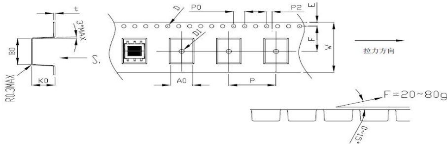
载带尺寸（TAPE DIMENSIONS）一般公差为±0.1mm
