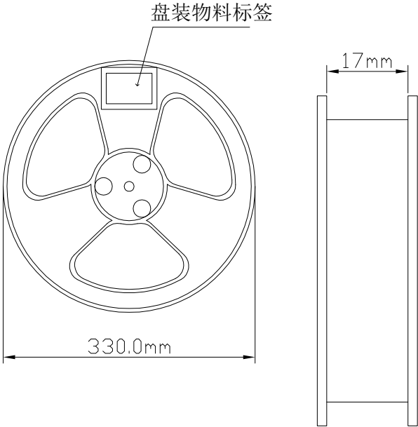
图3 盘装料盘
