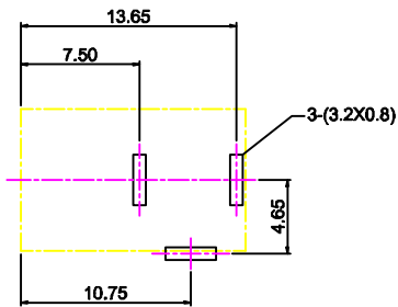
P.C.B 设计参考尺寸
