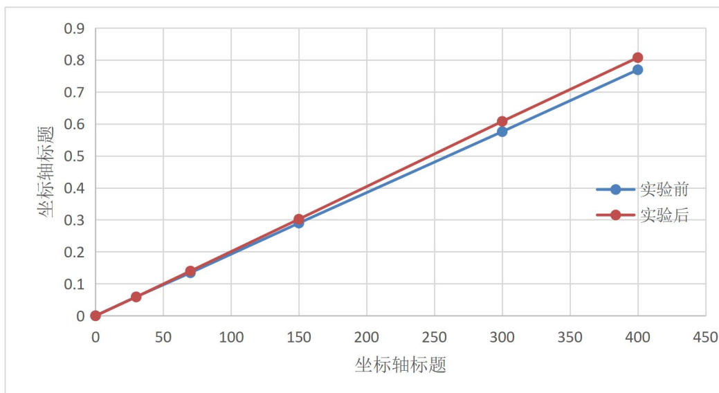
图 19 温度循环试验前后变化
