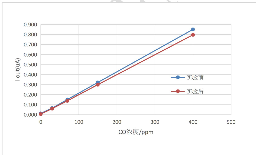
图 10 干扰气体试验前后测试变化
