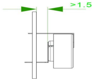
图 22 传感器与电路板焊接示意图
