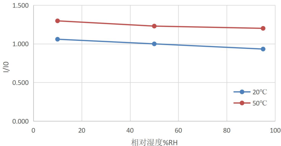
图 16 湿度影响
