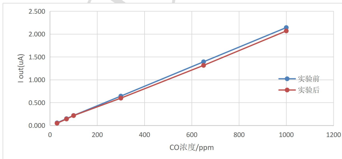
图 18 运输和储存试验前后变化
