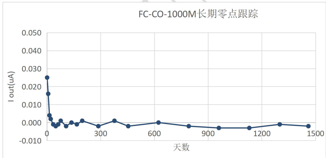
图 12 长期运行零点变化
