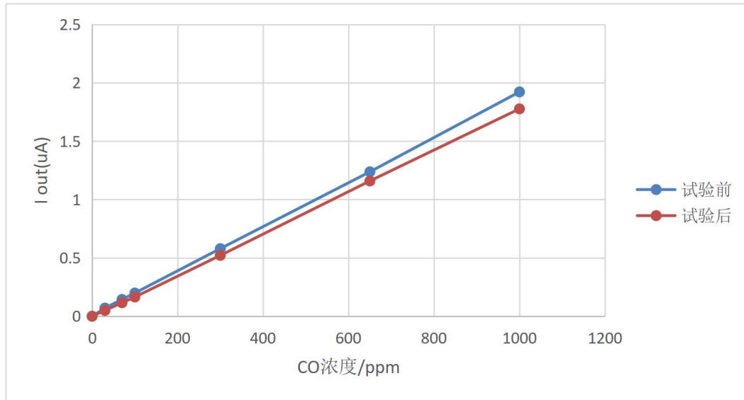
图 11 防腐性测试前后变化
