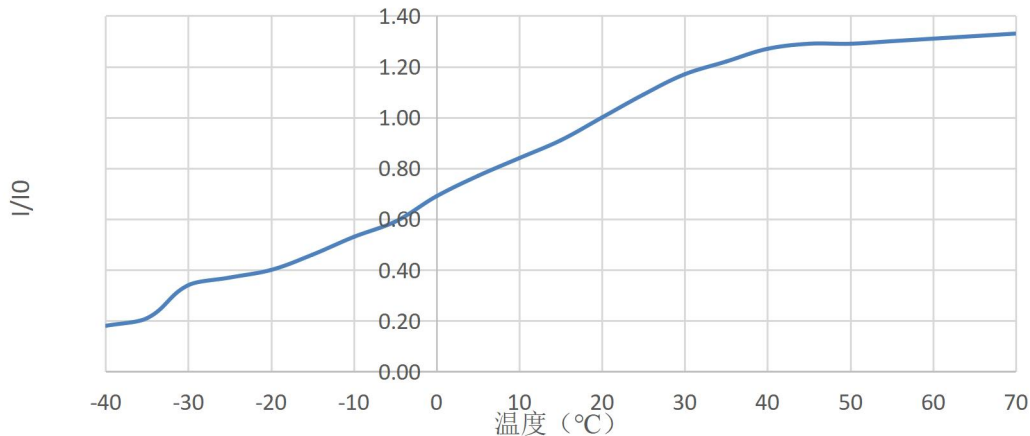
图 15 传感器温度补偿系数图示
