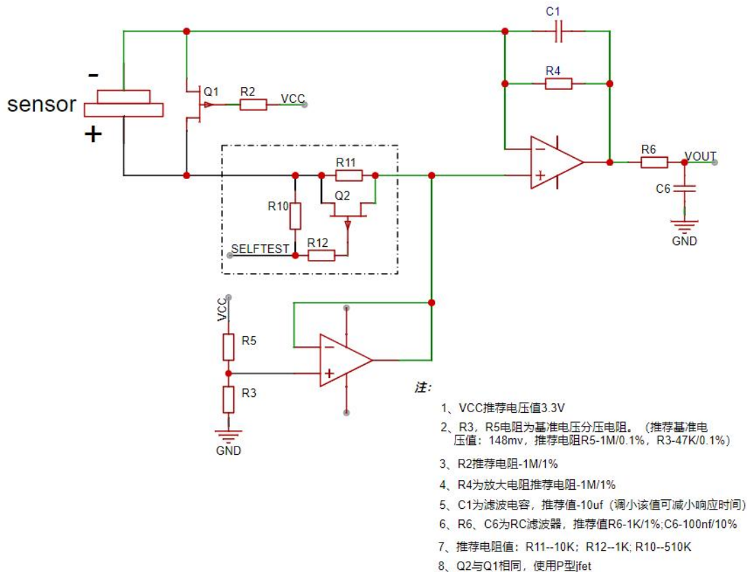
图 21 传感器电路示意图
