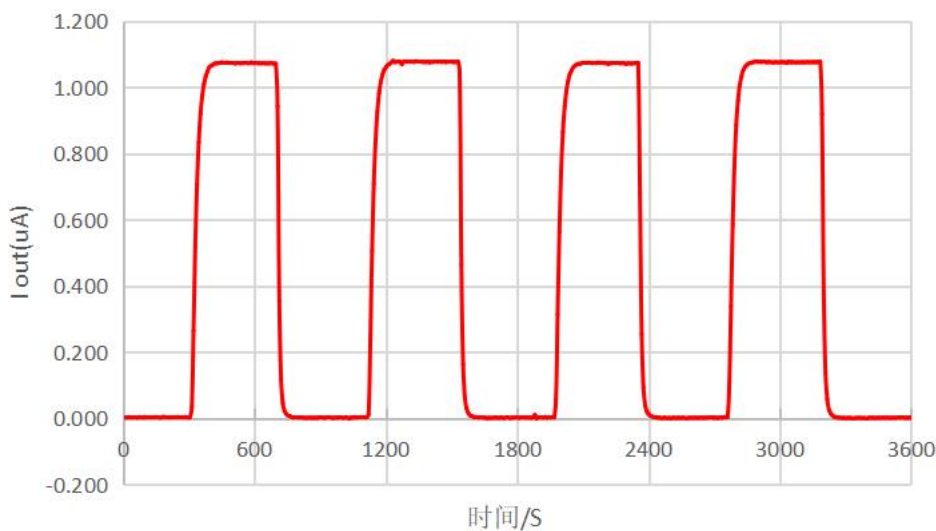
图 5 传感器对 500ppm 一氧化碳的重复性测试
