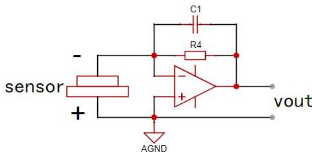
图 1 传感器基本测试电路
