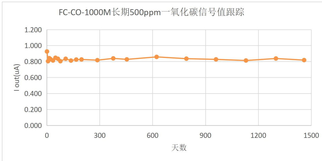
图 13 长期运行灵敏度变化
