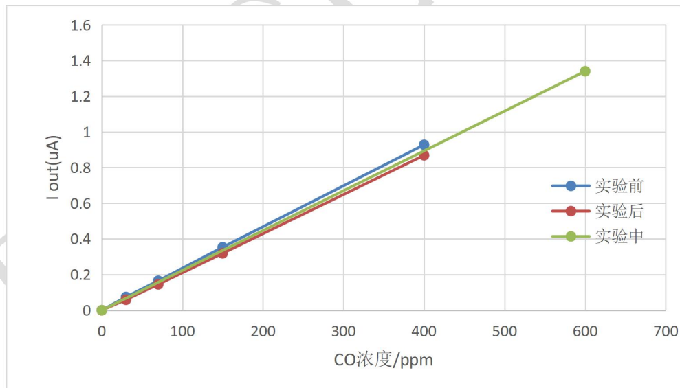
图 8 正常操作测试
