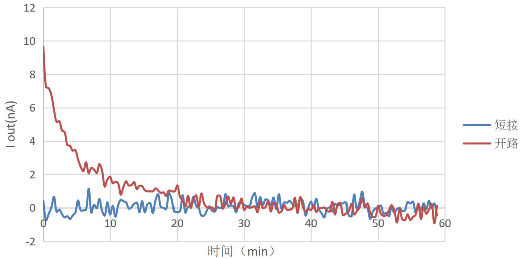
图 7 储存过程中短路和开路的影响
