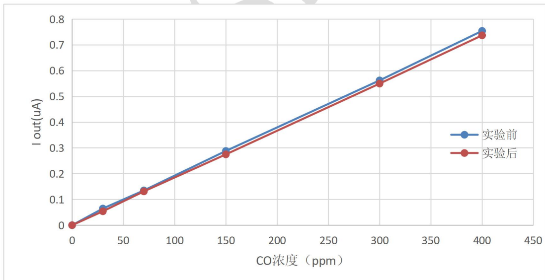
图 14 误报警测试
