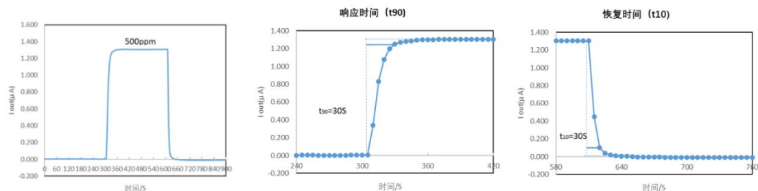
图 2 响应-恢复时间
