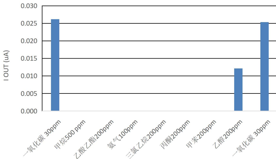
图 9 干扰耐久试验
