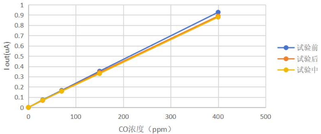
图 6 灵敏度试验前中后测试
