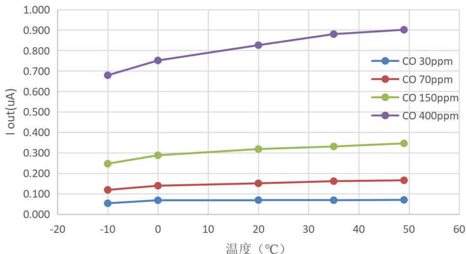
图 17 高低温运行试验
