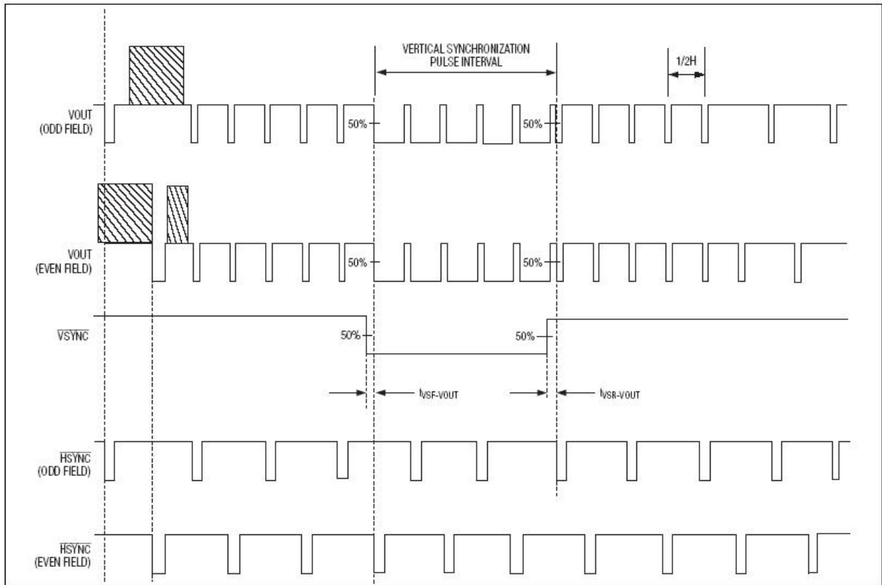
图7. VOUT、 \overline{\text{VSYNC}} 和HSYNC时序(PAL, 内同步模式)
