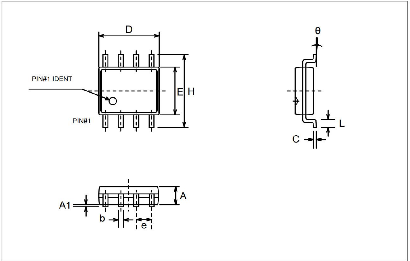
图 4-1: SOP8封装示例
