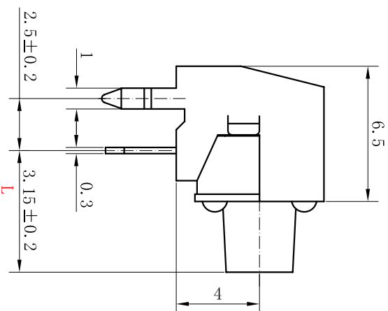
PCB线路板安装图(±0.1)
