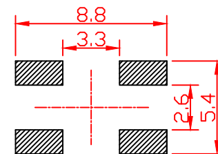
PCB. 焊接图
