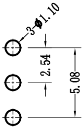
安装孔尺寸
