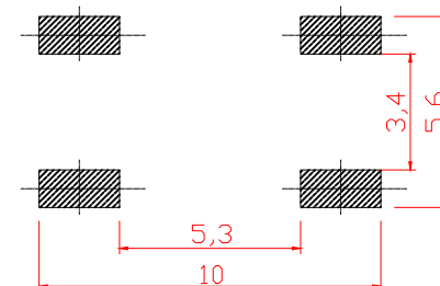
PCB. 焊接图
