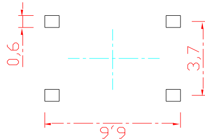
PCB. 焊接图
