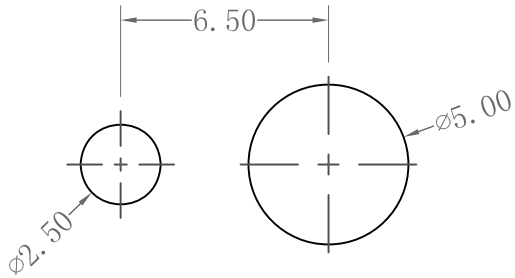
安装孔尺寸
