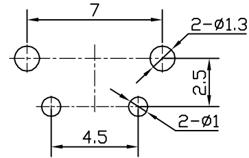
PCB线路板安装图( \pm 0.1 )
