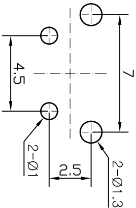
PCB线路板安装图(±0.1)
