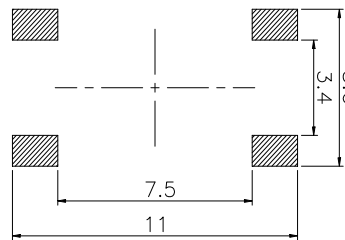
PCB. 焊接图
