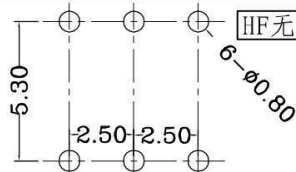
印刷电路板焊接处尺寸图
