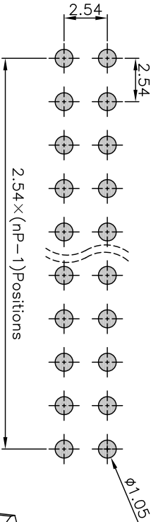
P.C.B LAYOUT
