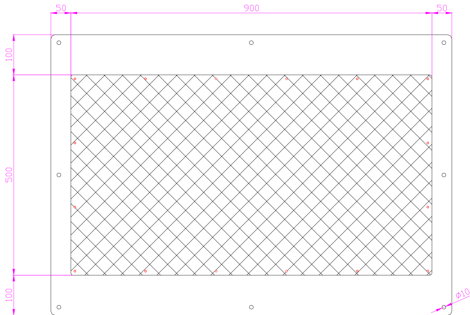
背面/侧面尺寸图
