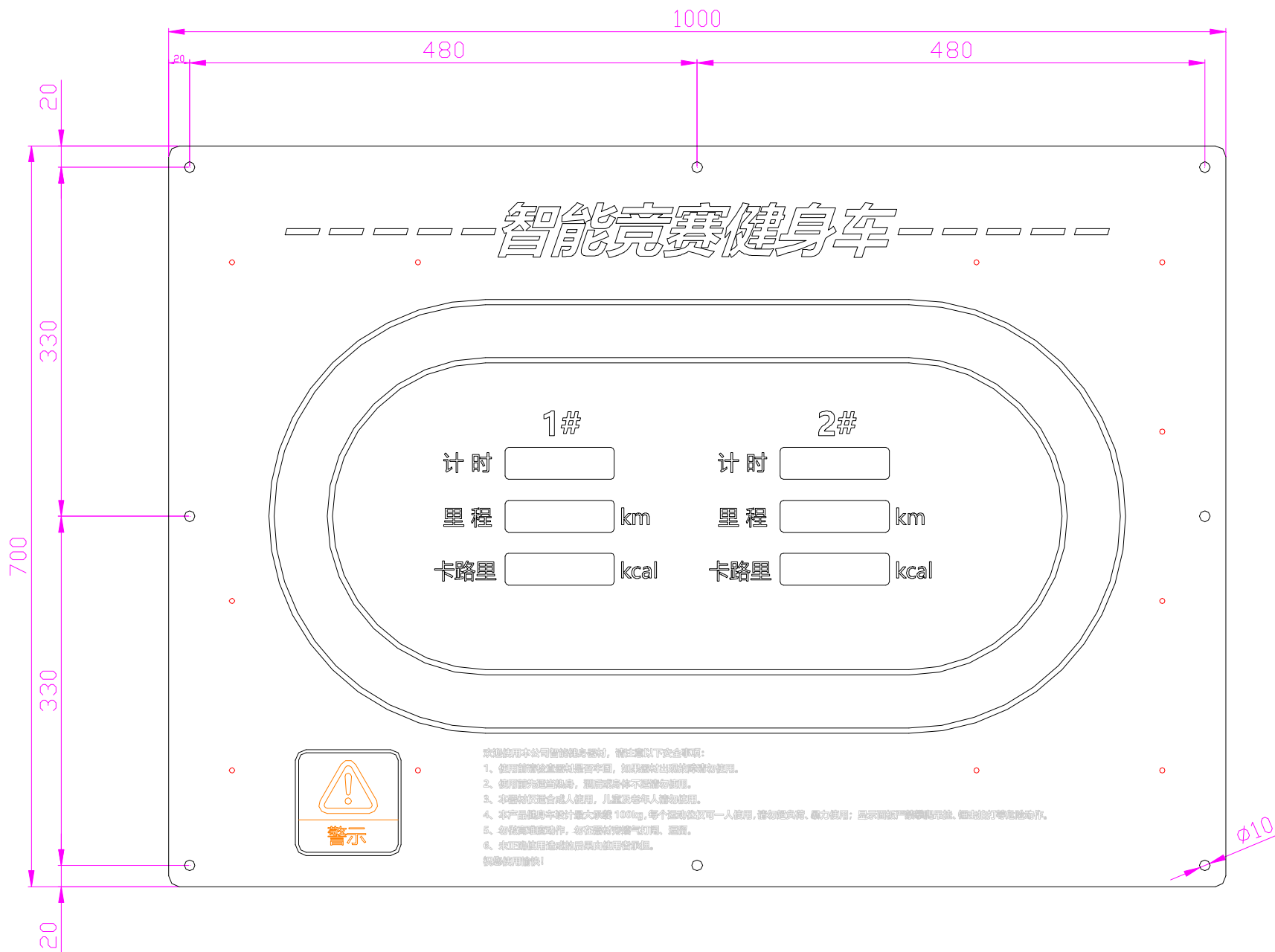
安装孔尺寸图
