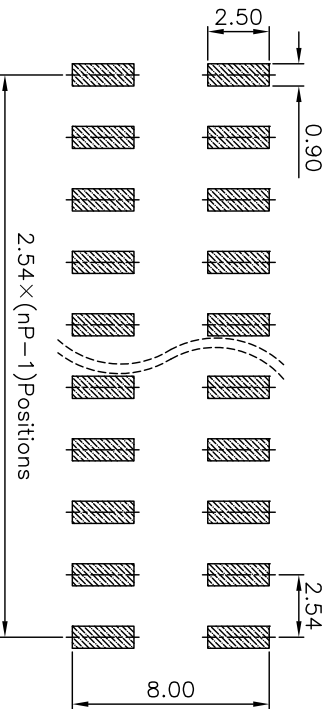
P.C.B LAYOUT
