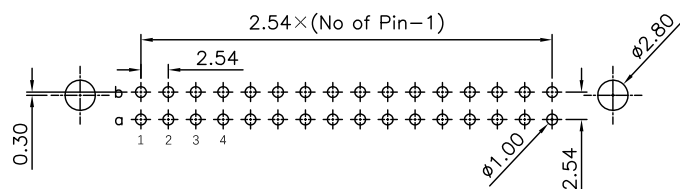
P.C.B LAYOUT
