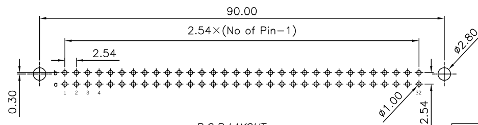
P.C.B LAYOUT
