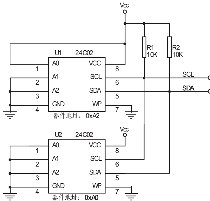
图15 EEPROM的级联
