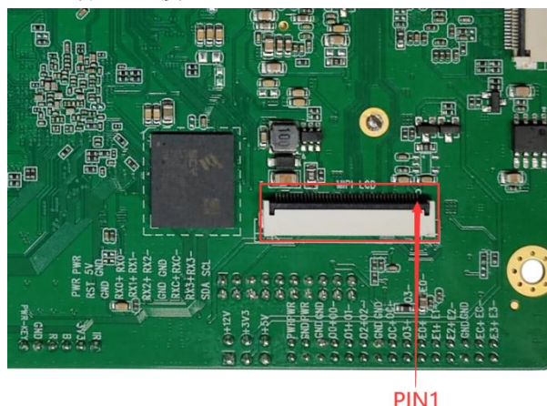
MIPI 屏 FPC 接口
