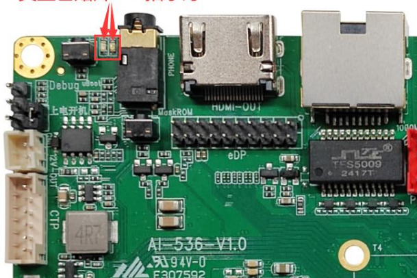
黄蓝色贴片LED指示灯
