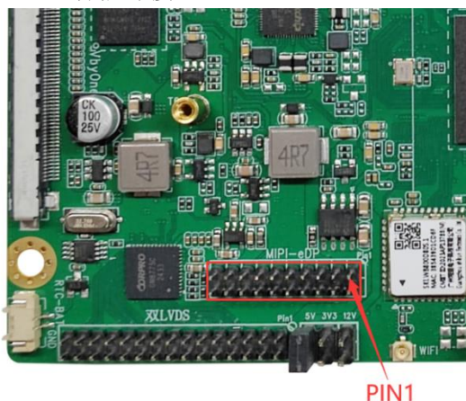
MIPI 屏插针接口
