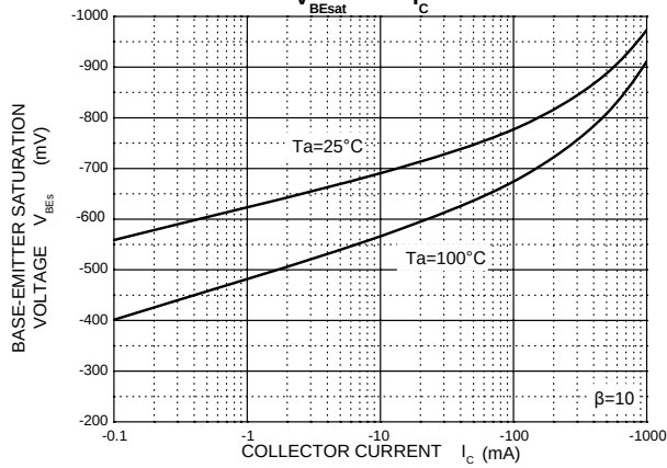
V_{BE} \text{ — } I_C
