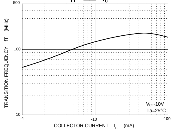
f_T \text{ — } I_C
